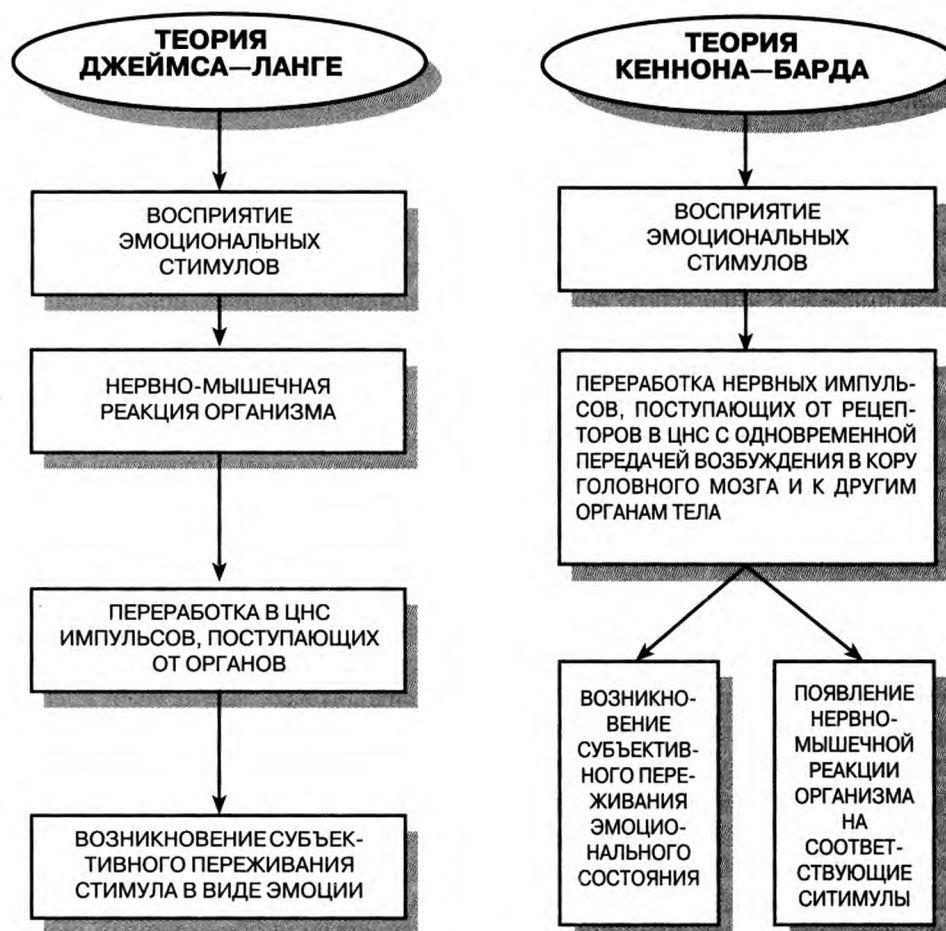
Рис. 16.2. Основные положения в теориях Джемса—Ланге и Кэннона—Барда
